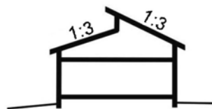
I Pulpettikatto 1:3
